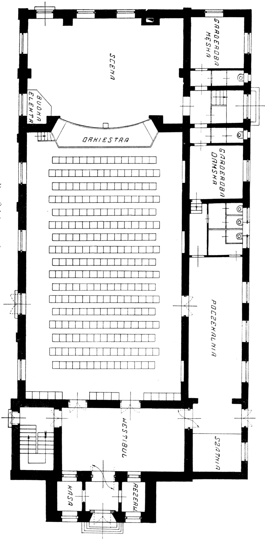
Dom Żołnierza w Łomży — rzut pionowy parteru.
